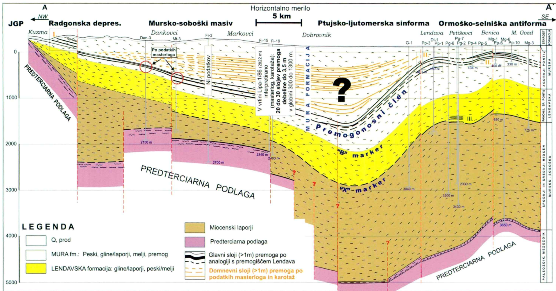
Sl. 17. Regionalni geološki prerez A-A' skozi Mursko-zalski bazen (horizontalno in vertikalno merilo je različno) (za potek glej sliko 16). Premoški »horizont« je prikazan shematično po analogiji s premogonosnimi plastmi na območju Lendava – Mursko Središče – Murski gozd (Prirejeno po MARIN-u et al. 1992). Podatki o izjemnem številu do 3,5 m debelih plasteh premoga obstajajo za vrtino Lipa-1, ki v projekciji na obravnavani prerez odgovarja približno situaciji v območju vrtin Filovci Fi-15 in Fi-19.
