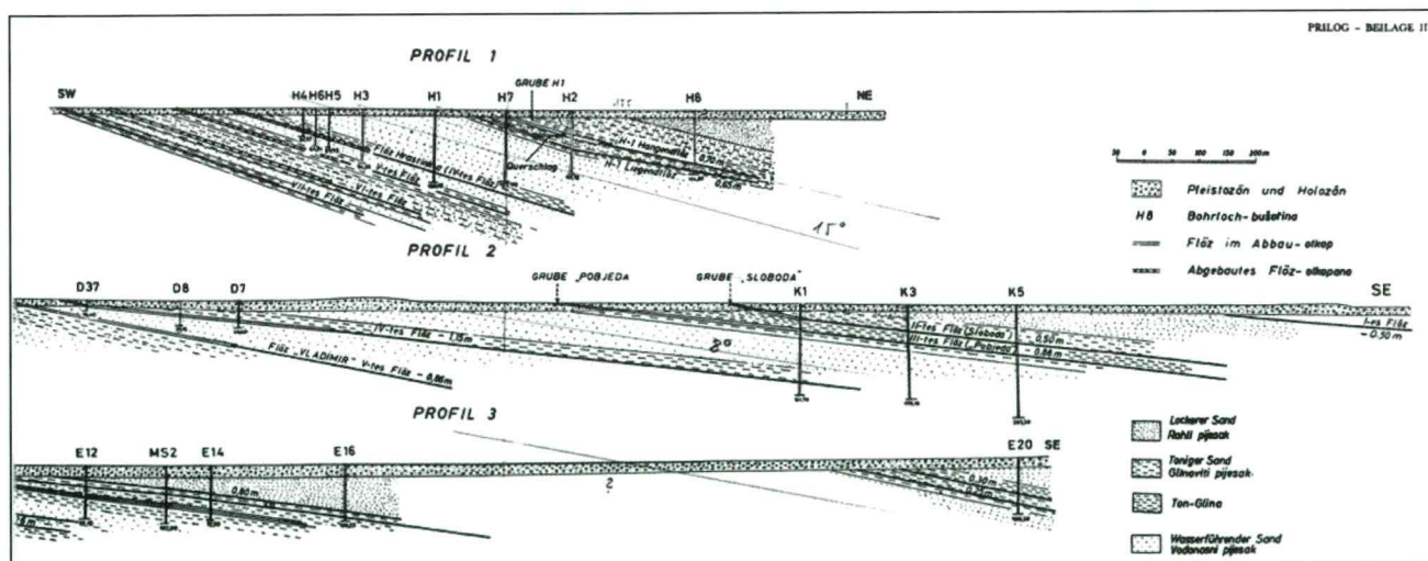
Sl. 10. Značilni geološki prerezi premogišča Mursko Središče (Takšić, 1967).
