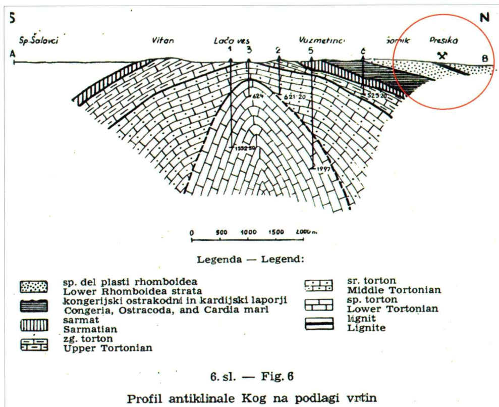
Sl. 6. Geološki prerez (na podlagi podatkov iz vrtin »Kog«) skozi Ormoško-selniško antiformo (antiklinalo Kog) v smeri od Pesike na severu (glej sliko 5) proti jugu (kopirano iz PLENIČAR, 1954).
