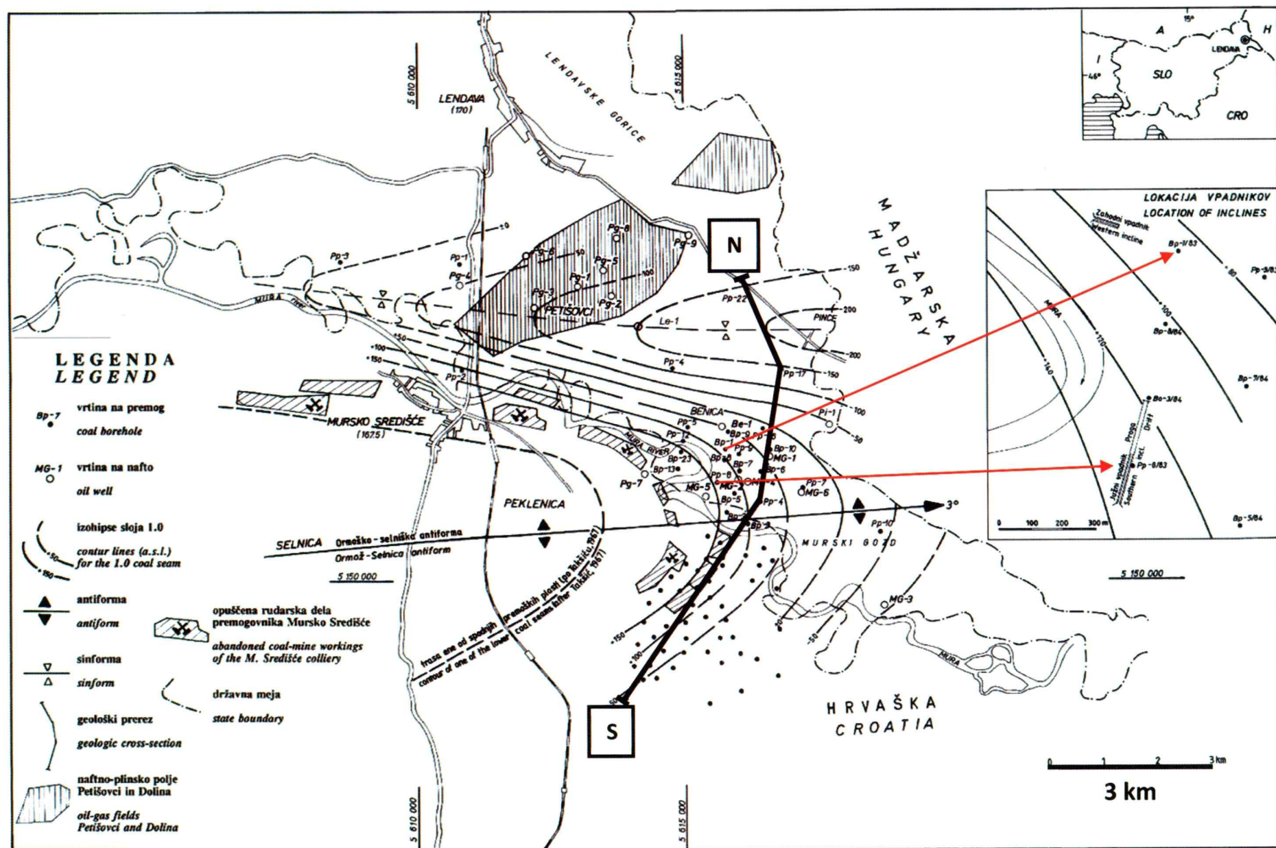
Sl. 12. Strukturna karta premogovih plasti (za sloj 1.0) na območju med Lendava – Mursko Središće – Murski gozd (MARKIĆ & GRAD, 1991).
