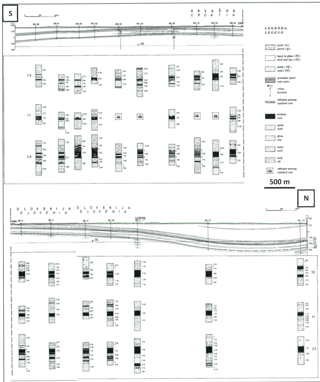
Sl. 13. Geološki prerez premogonosnih plasti na območju Lendava – Mursko Središče (označen na karti na sliki 12) od juga (zgoraj levo) proti severu (spodaj desno). Po podatkih iz vrtin so podrobno prikazani stolpci glavnih treh slojev premoga (1.0, 1.1 in 2.0) z njihovo neposredno talnino in krovino (MARIN et al., 1989a).
