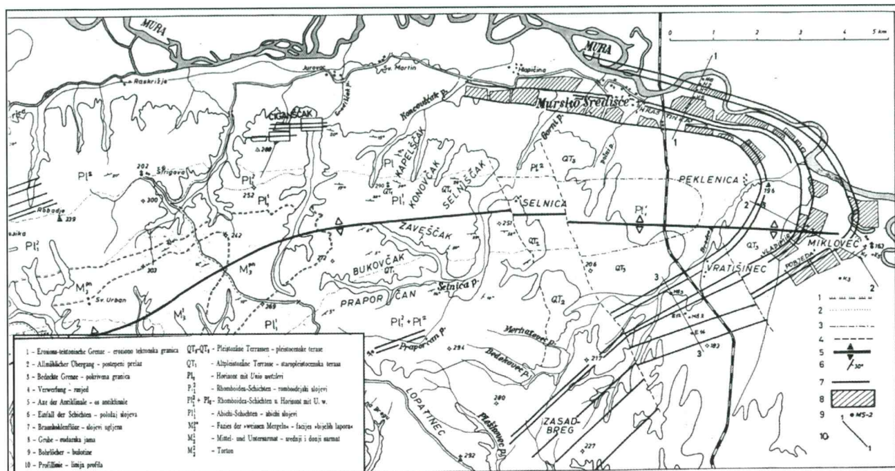
Sl. 9. Strukturna karta premogišča Mursko Središče (Takšić, 1967).
