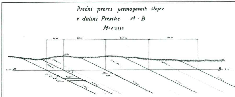
Sl. 7. Lega slojev premoga in rudarska dela v premogišču Presika (KARNIČNIK, okoli leta 1965 ?). Prerez poteka približno od juga (A) proti severu (B) (op.p.) Nagib plasti je 25°. Globina najglobljšega rudarskega dela je okoli 100 metrov pod površino.
