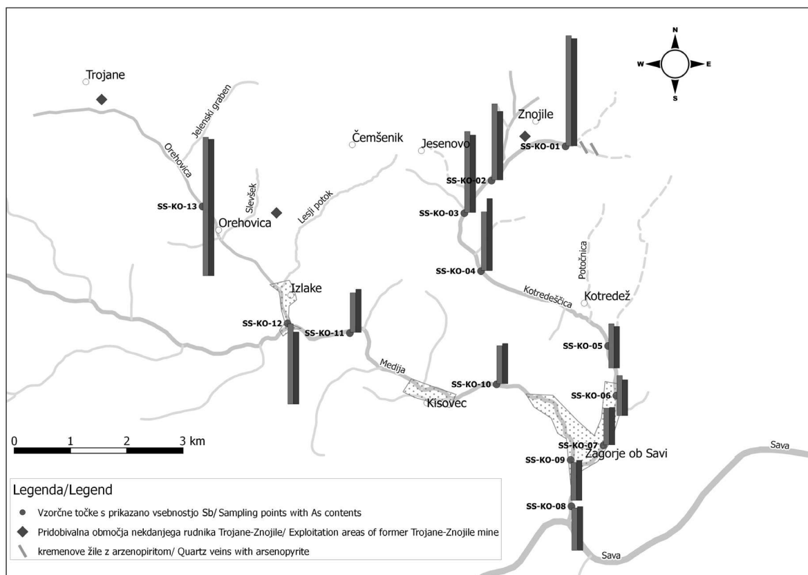
Sl. 6. Prikaz vzorčnih mest in vsebnosti antimona (Sb) v mg/kg v vzorcih sedimentov na vplivnem območju Kotredešice (levi stolpci prikazujejo vsebnost Sb v frakciji <0,125 mm, desni v frakciji <0,063 mm).
