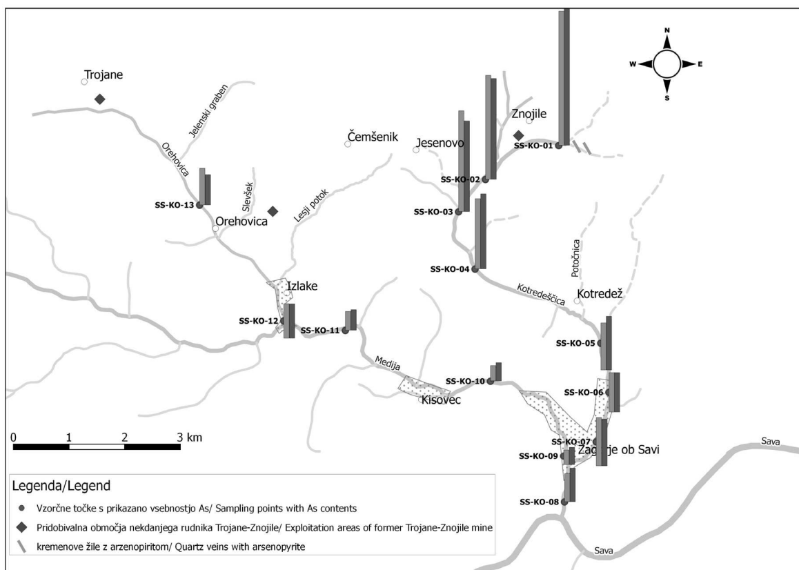
Sl. 5. Prikaz vzorčnih mest in vsebnosti arsena (As) v mg/kg v vzorcih sedimentov na vplivnem območju Kotredešice (levi stolpci prikazujejo vsebnost As v frakciji <0,125 mm, desni v frakciji <0,063 mm).
