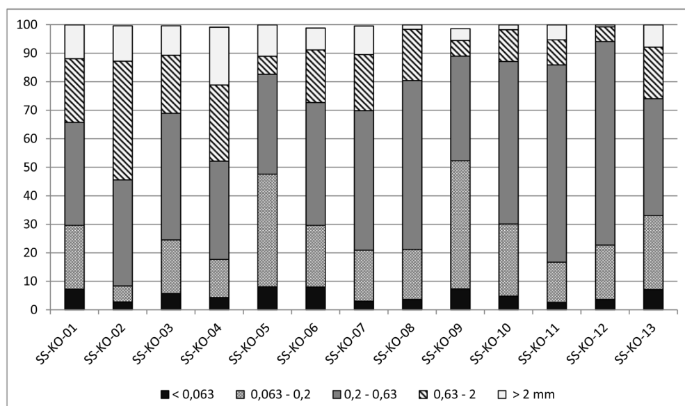
Sl. 4. Razmerje deležev proda, debelo, srednje in drobnnozrnatega peska ter mulja v vzorcih sedimentov.
