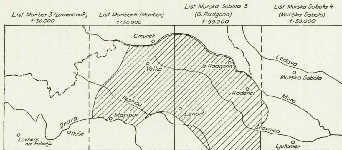
Pregled kartiranega ozemlja na listih Maribor in Murska Sobota (1 : 100.000)
