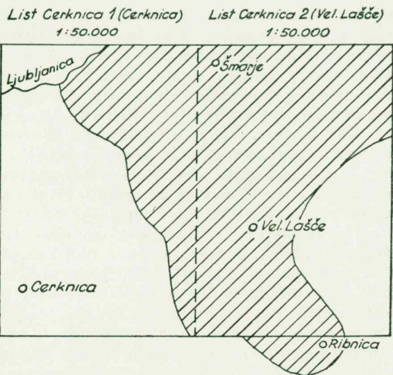
Pregled kartiranega ozemlja na listu Cerknica (1 : 100.000)
