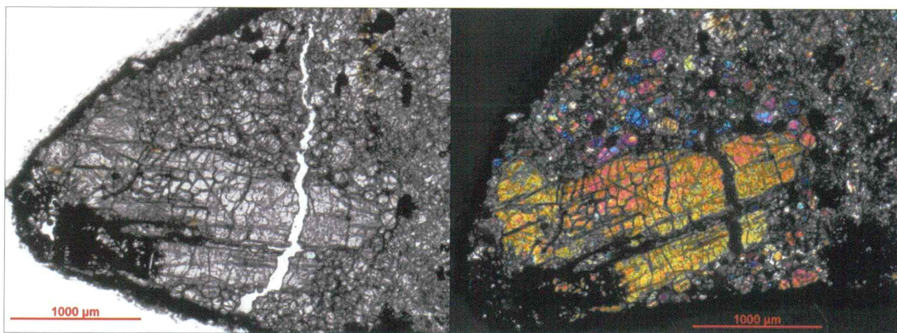
Sl. 17. Porfirna olivinova hondrula z reliktnim zrnem olivina. Presevna polarizirana svetloba, || nikoli (levo), x nikoli (desno).
