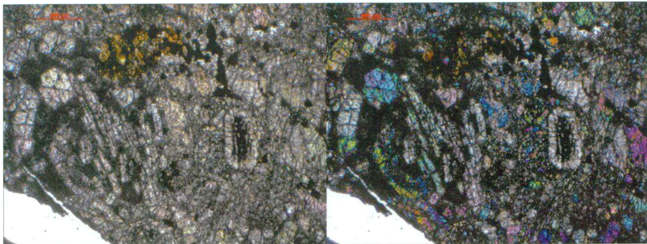
Sl. 5. Meteorit Jesenice. Številne zelo rekristalizirane olivinove hondrule. Presevna polarizirana svetloba, || nikoli (levo), x nikoli (desno).
