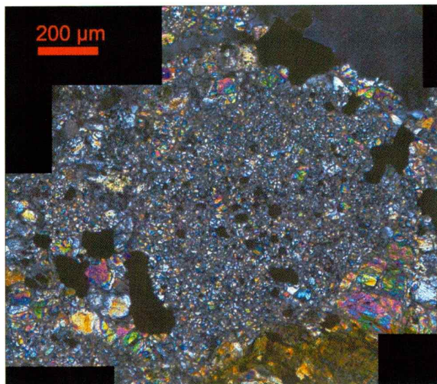
Sl. 14. Meteorit Jesenice. Zrnata olivinova-piroksenova hondrula. Zrna olivina in piroksena so dovolj velika, da jih z optičnim mikroskopom prepoznamo. Velikost zrn se proti robu hondrule povečuje. Presečna polarizirana svetloba, x nikoli.
