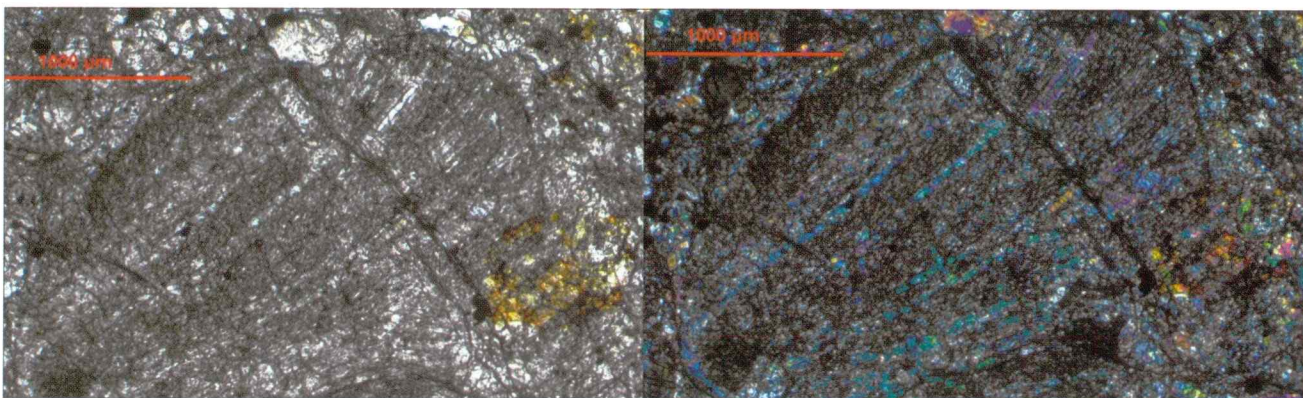
Sl. 10. Meteorit Jesenice. Pahljačasta piroksenova hondula. Drobnna piroksenova zrna rastejo usmerjeno iz skupne nukleacijske točke. Siva zelo drobnnozrnata osnova ima sestavo glinencev. Presečna polarizirana svetloba, || nikoli (levo), x nikoli (desno).
