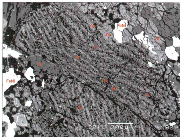
Sl. 13. Meteorit Jesenice. Polisomatska lamelarna olivino-va hondrula je zgrajena iz podolgovatih zrn olivina (Ol) in plagiklaza (Pl) ter iz železovo-nikljevih mineralov (FeNi) v različnih orientacijah. SEM, BSE.
