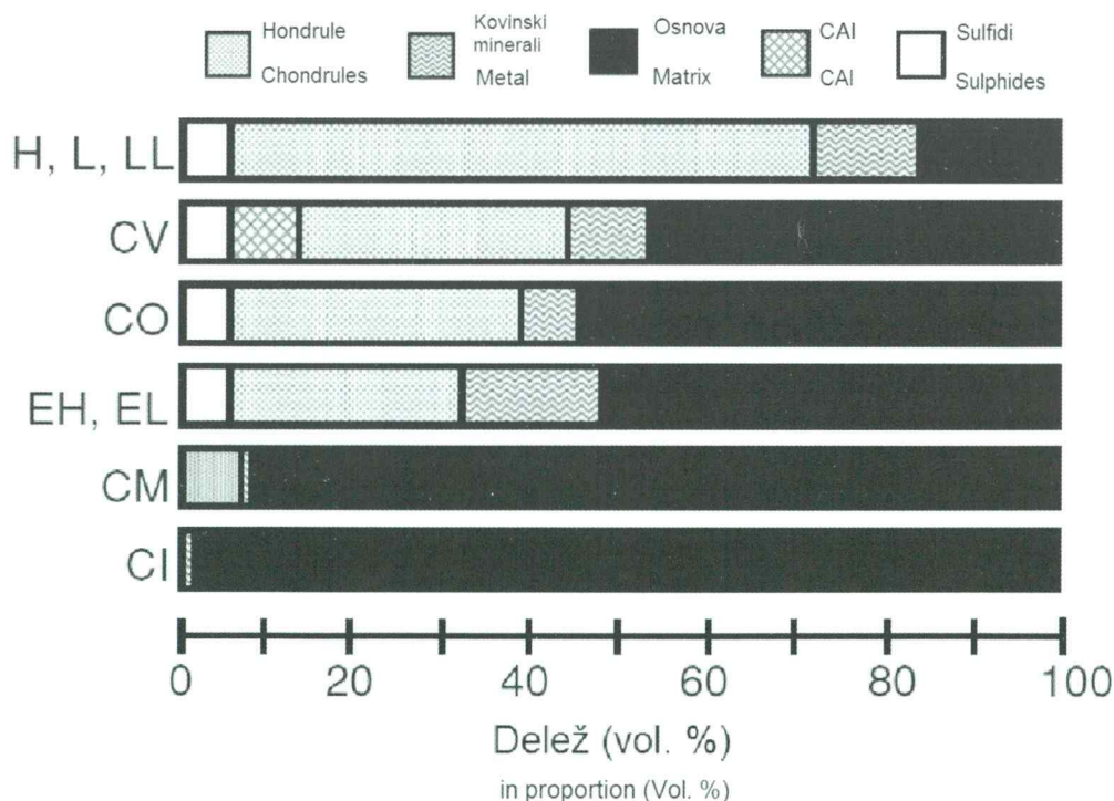
Sl. 4. Povprečna sestava različnih vrst hondritov (povzeto po SEARS, 2004)
