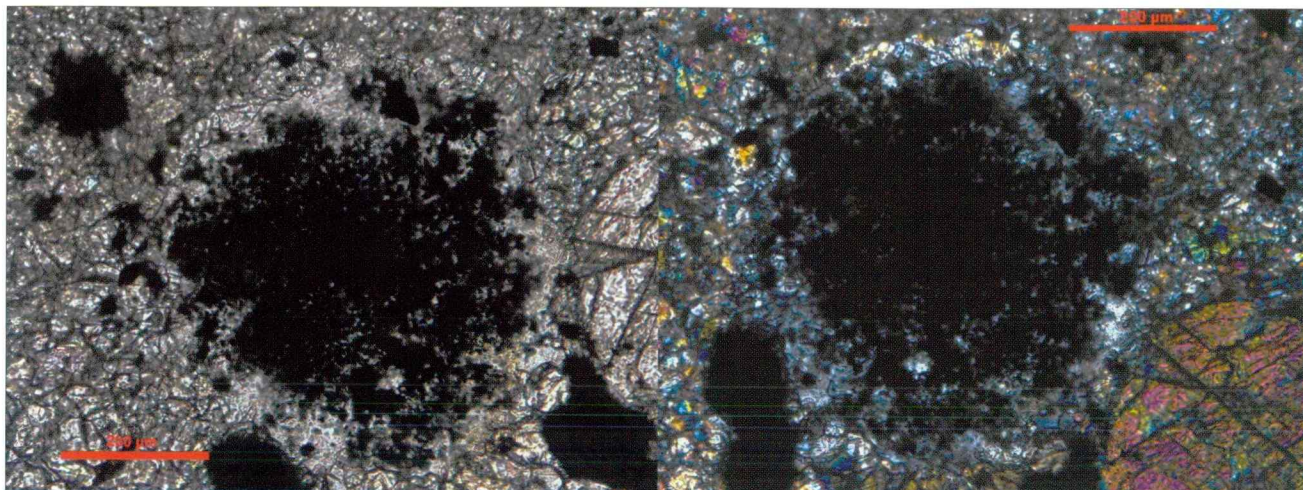
Sl. 15. Meteorit Jesenice. Kovinska hondrula. Središče hondrule je sestavljeno predvsem iz drobnih zrn nepresevnih železovo-nikljevih mineralov. Skorjico oblikujejo zrna glinenec. Presevna polarizirana svetloba, || nikoli (levo), x nikoli (desno).
