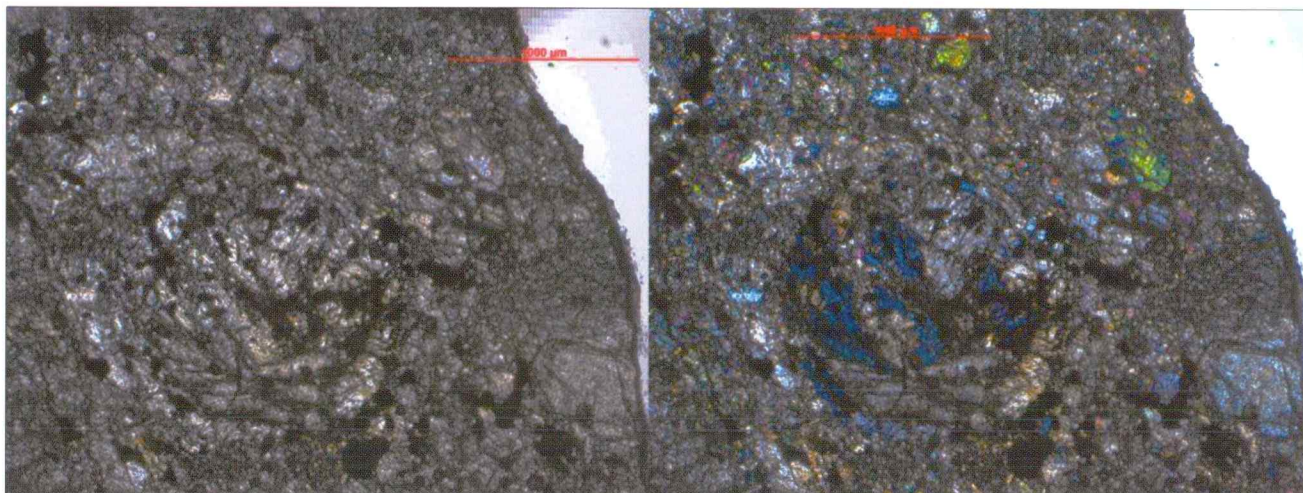
Sl. 9. Meteorit Jesenice. Porfirna piroksenova hondula. Presečna polarizirana svetloba, || nikoli (levo), x nikoli (desno)
