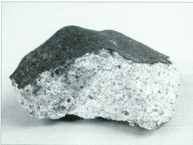
Sl. 1. Meteorit Jesenice. Rumeno-rjave lise so sekundarni železovi minerali, ki so posledica oksidacije železovih mineralov. Črni sloj je žgalna skorja meteorita.
