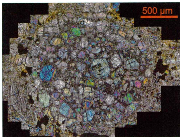
Sl. 7. Meteorit Jesenice. Porfirna olivinova hondrula. Hondrulo sestavljajo evhedralna do subehedralna zrna olivina, poplajena v drobnozrnatni osnovi. Presevna polarizirana svetloba, x nikoli.
