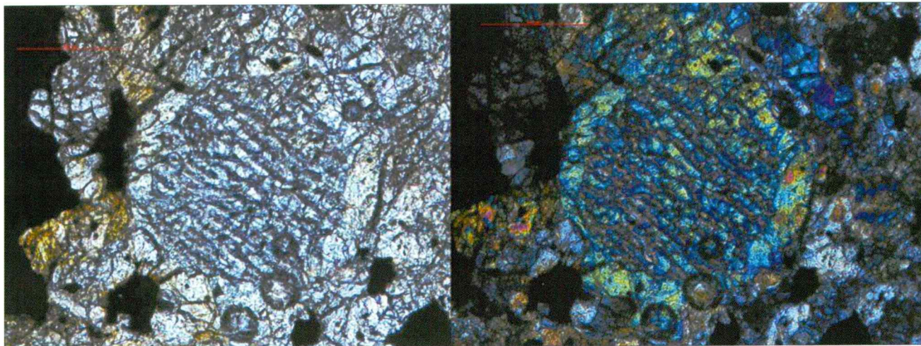
Sl. 12. Meteorit Jesenice. Lamelarna olivinova hondrula z debeložrnato skorjico. Presečna polarizirana svetloba, || nikoli (levo), x nikoli (desno).
