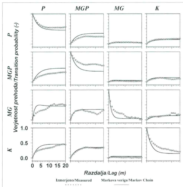
Slika 3. Verjetnosti prehodov v vertikalni (z) smeri (meritve in model Markovih verig)
