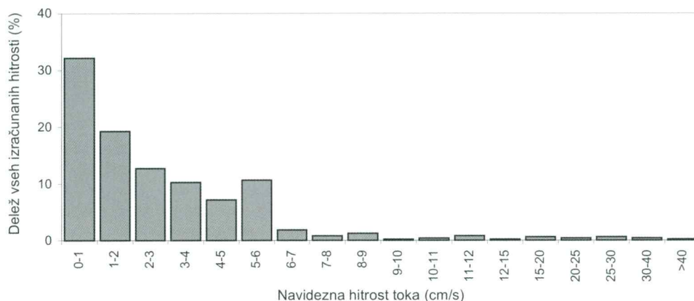
Sl. 3. Razporeditev izračunanih navideznih hitrosti podzemnega pretakanja Fig. 3. Distribution of calculated apparent groundwater flow velocities
