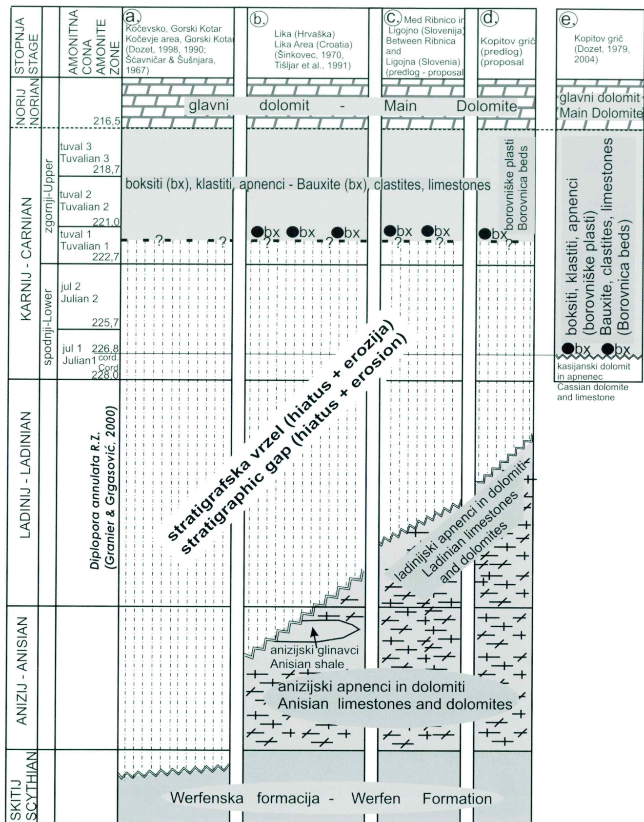
Slika 2. Stratigrafska primerjava triasnih razvojev v osrednji Sloveniji in Liki na Hrvaškem, s posebnim poudarkom na karnijski prekinitvi morske sedimentacije. Karnijska conacija na podlagi OGG (2004), starosti v milijon letih. a.) Kočevsko, Gorski Kotar (DOZET 1998, 1990; ŠČAVNIČAR & ŠUŠNJAR, 1967); b.) Lika (Hrvaška) (ŠINKOVEC, 1970; TIŠLIJAR et al., 1991); c.) Osrednja Slovenija (predlog – ta prispevek); d.) Kopitov grič (predlog – ta prispevek); e.) Kopitov grič (DOZET, 1979, 2004). Figure 2. Stratigraphical correlation of Triassic developments in the Central Slovenia and Lika in Croatia, with emphasis on the Carnian break of the marine sedimentation. Carnian zonation based according to OGG (2004), ages in million years. a.) Kočevsko, Gorski Kotar regions (DOZET 1998, 1990; ŠČAVNIČAR & ŠUŠNJAR, 1967); b.) Lika region (Croatia) (ŠINKOVEC, 1970; TIŠLIJAR et al., 1991); c.) Central Slovenia (proposal – this work); d.) Kopitov grič locality (proposal – this work); e.) Kopitov grič locality (DOZET, 1979, 2004).
