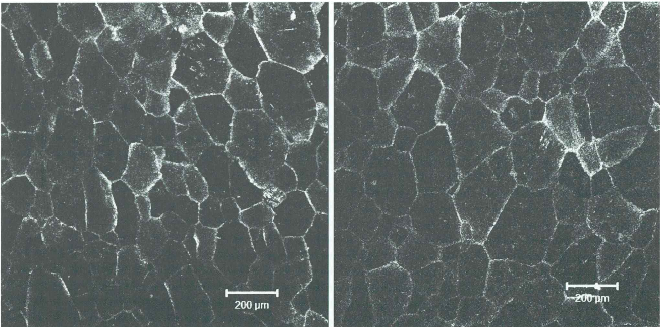
Slika 3 (levo) in slika 4 (desno). 2D posnetek mikrostrukture svežega (levo) in staranega (desno) kalcitnega marmorja. V obeh primerih prevladujejo plitve razpoke med zrn, kar je vidno tudi iz intenzitete razpok na slikah (nimajo »odebeljenih« robob). Posnetka sta narejena s plan-akromatskim objektivom (povečava objektivna 10 x; 0,45 NA).
