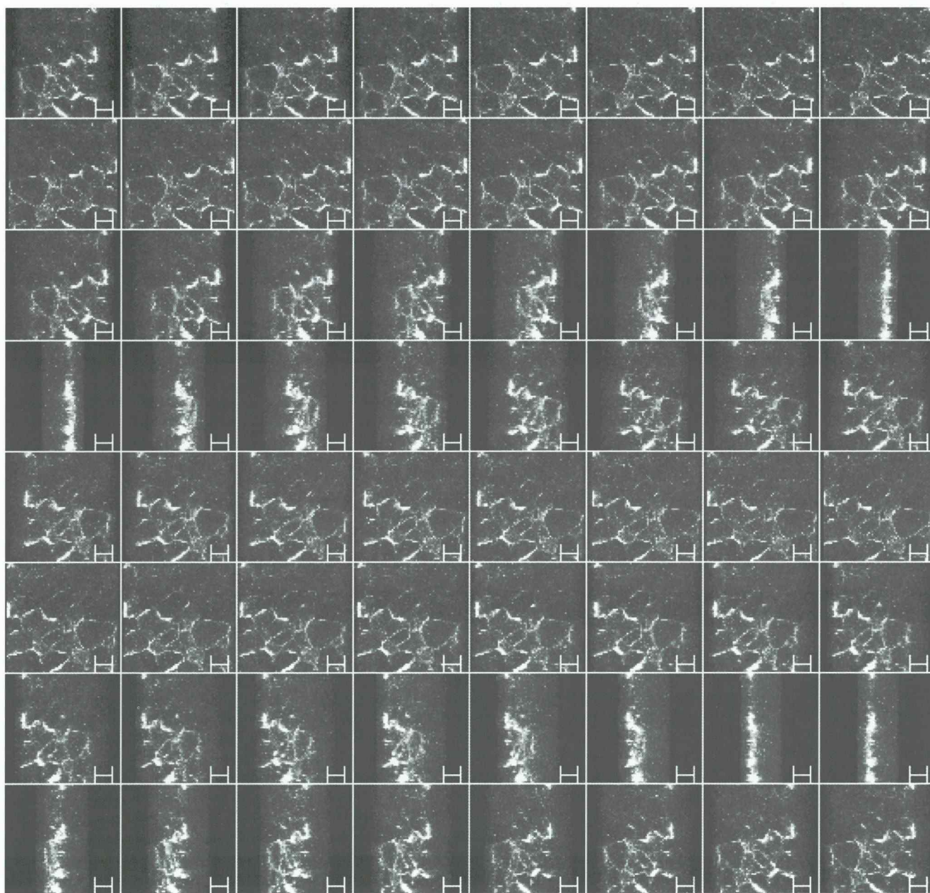
Slika 7. Galerija posameznih faz projekcije staranega vzorca po 104 ciklih zmrzovanja in tavanja. Posamezne sličice gledano od leve proti desni predstavljajo v tem primeru optično rezino, rotirano okrog x-y osi (povečava objektiva 10x; 0,45 NA, velikost enega kvadrata je 1371,72 x 1303,00 \mu\text{m} )
