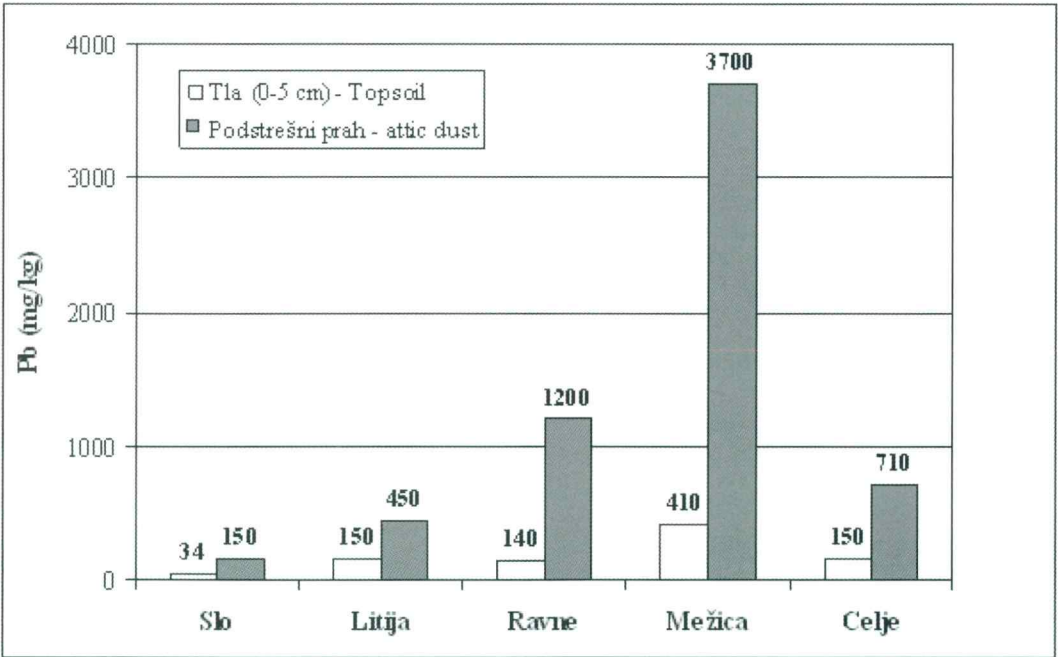
Slika 5. Vsebnosti Pb v tleh in podstrešnem prahu na območju Slovenije, Litije, Raven na Koroškem, Mežici in Celju. Figure 5. Pb concentrations in topsoil and attic dust in areas of Slovenia, Litija, Ravne na Koroškem, Mežica and Celje.
