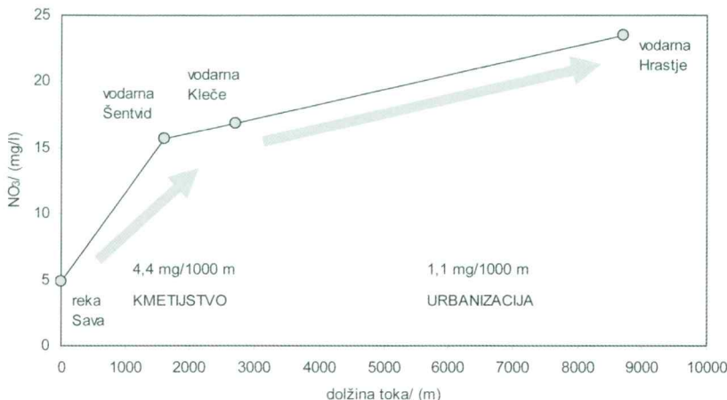
Slika 9. Koncentracije nitrata vzdolž toka podzemne vode preko vodarne Kleče do vodarne Hrastje.
