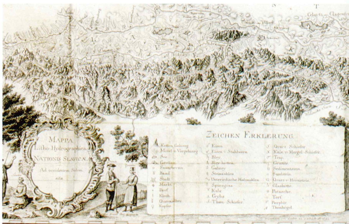
Sl. 2. Hacquetova Mappa Litho-Hydrographica Nationis Slavicae Ad occidentem Solem sitae (Litohidrografska karta južnozahodnega slovanskega ozemlja, 1784). Ni v merilu.
