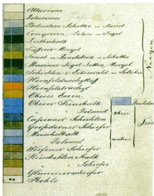
Sl. 4. Del Lipoldove karte Motnik in Celje (1854–1856), M 1 : 144 000.
