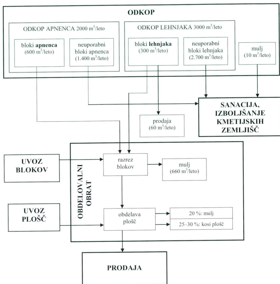
Slika 2. Snovni tok apnenca in lehnjaka v Marmorju Hotavlje d.d.
