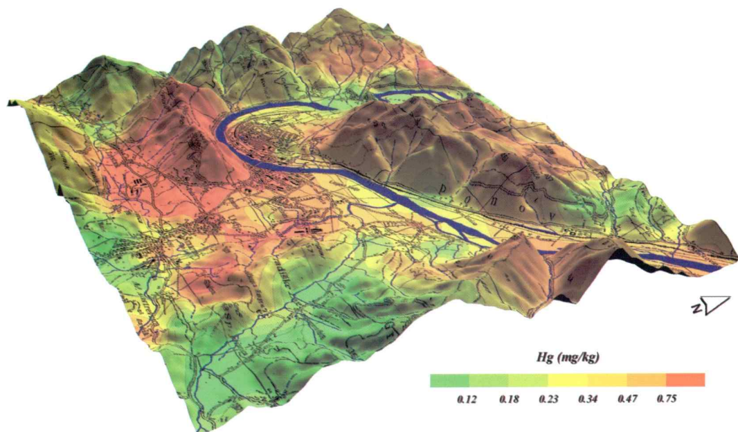
Slika 8a. Porazdelitev živega srebra v zgornjem horizontu tal (0–5 cm)
