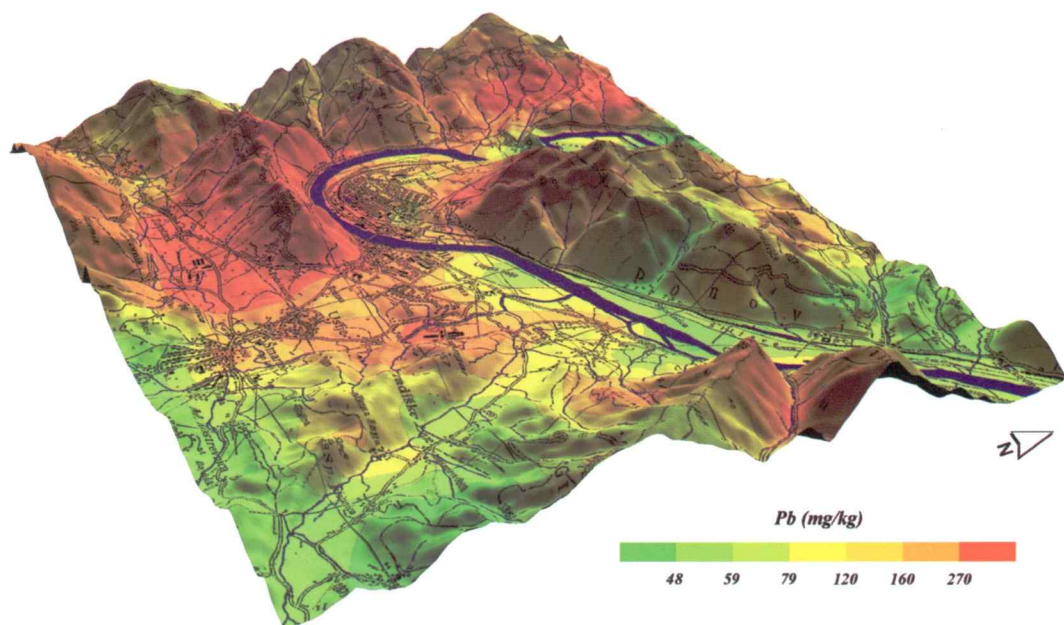
Slika 9a. Porazdelitev svinca v zgornjem horizontu tal (0–5 cm)
