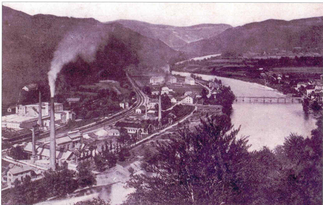
Slika 4. Topilnica svinca v Litiji leta 1910
