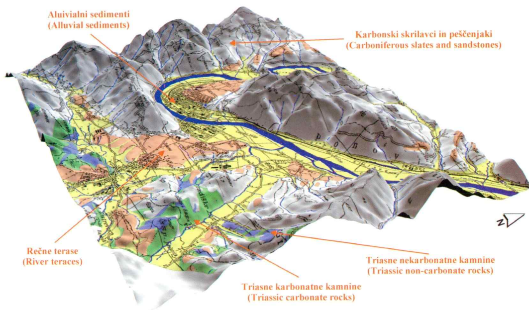
Slika 2. Pregledna geološka karta raziskanega ozemlja
