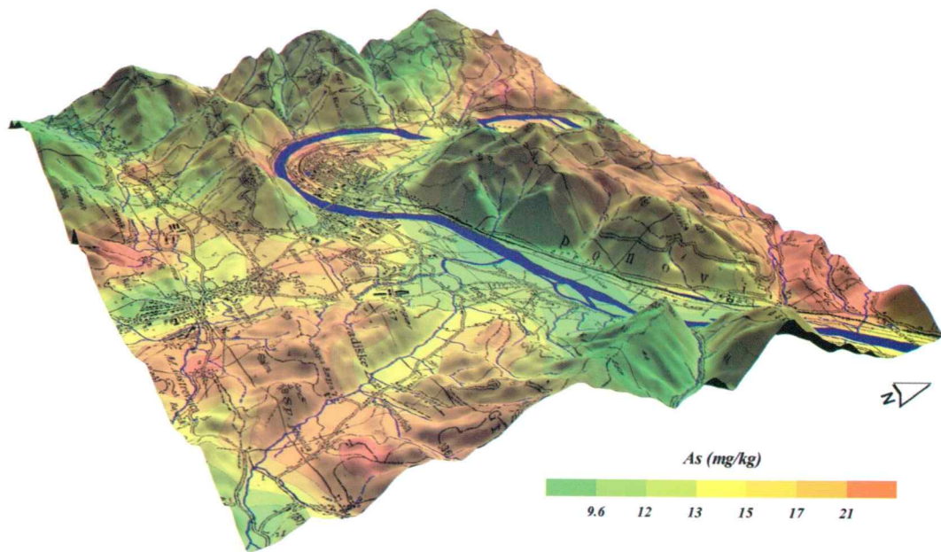
Slika 7b. Porazdelitev arzena v spodnjem horizontu tal (20–30 cm)
