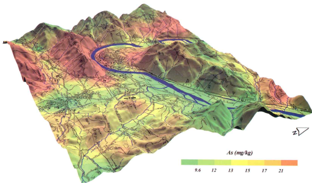
Slika 7a. Porazdelitev arzena v zgornjem horizontu tal (0–5 cm)
