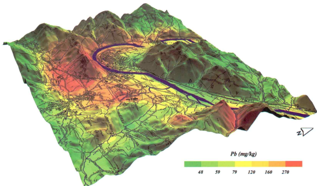
Slika 9b. Porazdelitev svinca v spodnjem horizontu tal (20–30 cm)
