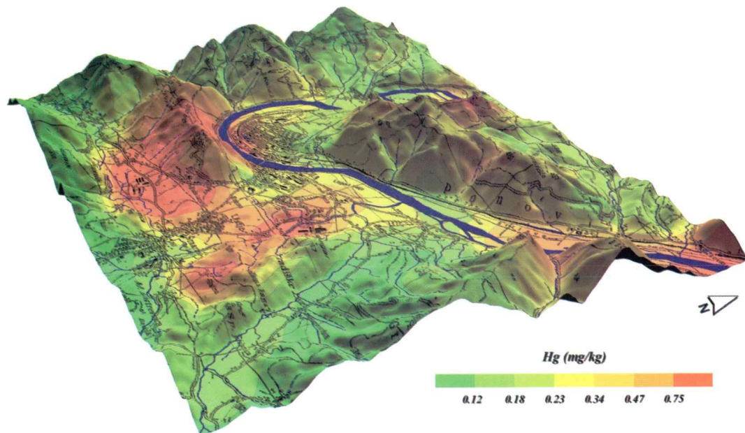
Slika 8b. Porazdelitev živega srebra v spodnjem horizontu tal (20–30 cm)
