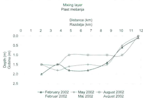
Slika 2. Globina plasti mešanja sladke in slane vode v estvarju reke Soče
