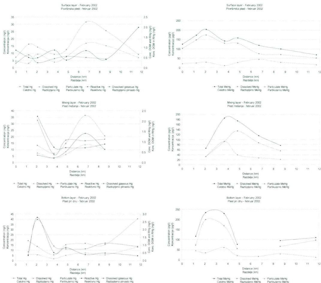
Slika 3. Dolvodna razporeditev različnih Hg oblik v različnih plasteh vodnega stolpca februarja 2002
