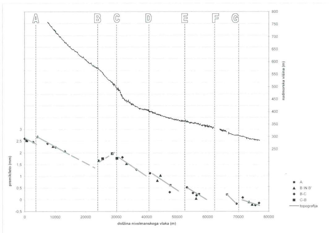
Sl. 3. Primerjava topografskega profila Save in podatkov nivelmanskega vlaka (projekcija na vertikalno ravnino s slemenitvijo 128°). Nakazana je segmentacija profila na osem odsekov. Oznake A, B in B', B-C in C-B so kategorije reperjev glede na geološko podlago in kvaliteto vgradnje.
