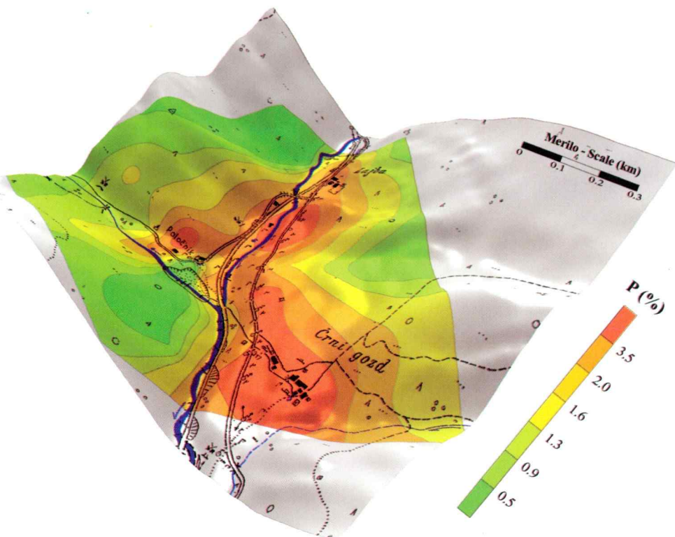
Sl. 6. Porazdelitev fosforja v tleh (0-5cm).
