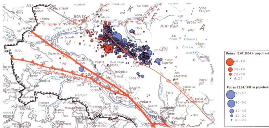
Slika 5. Epicenter glavnega potresa in popotresnih sunkov 12. aprila 1998 (modri krogci) in zadnjega potresa 12. julija 2004 (rdeči krogci). Velikost krogcev opredeljuje magnitudo.
