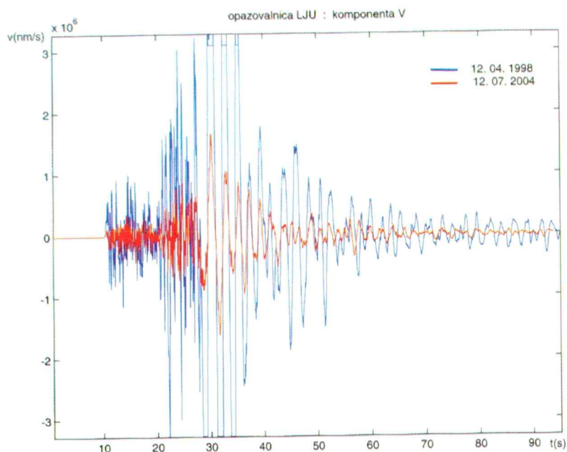
Slika 4. Primerjava zapisov potresov 12. aprila 1998 (modri seizmogram) in 12. julija 2004 (rdeči seizmogram) nam nazorno kaže, da je bil zadnji potres po sproščeni energiji bistveno šibkejši.
