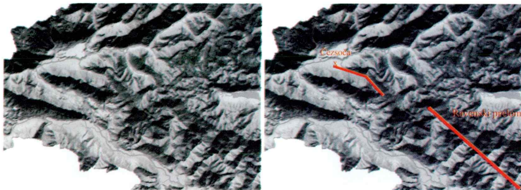
Slika 8. Reliefna karta zg. Posočja DMR (levo) in potek lepo vidnega Ravenskega preloma, ter prečnega preloma, ki poteka čez vas Čezsočo (desno), ob katerem sta nastala potresa 12. aprila 1998 in 12. julija 2004.
