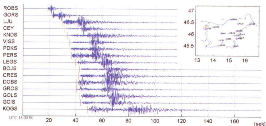
Slika 3. Zapisi glavnega potresa 12. julija 2004 na delujočih opazovalnicah državne mreže potresnih opazovalnic (ROBS-Robič pri Kobaridu, GORS-Gorjuše na Pokljuki, LJU-Golovec v Ljubljani, CEY-Goričice ob Cerkljanskem jezeru, KNDS-Knežji dol nad Ilirsko Bistrico, VISS-Višnje, PDKS-Podkum, PERS-Pernice, LEGS-Legarje, BOJS-Bojanci v Beli krajini, CRES-Črešnjevec, DOBS-Dobrina, GROS-Grobnik na Pohorju, GOLS-Goliše, GCIS-Gornji Cirknik, KOGS-Kog). Rdeča črta kaže prihod primarnih valov, zelena pa sekundarnih, avtomatski izračun epicentra pa je na sliki desno zgoraj.
