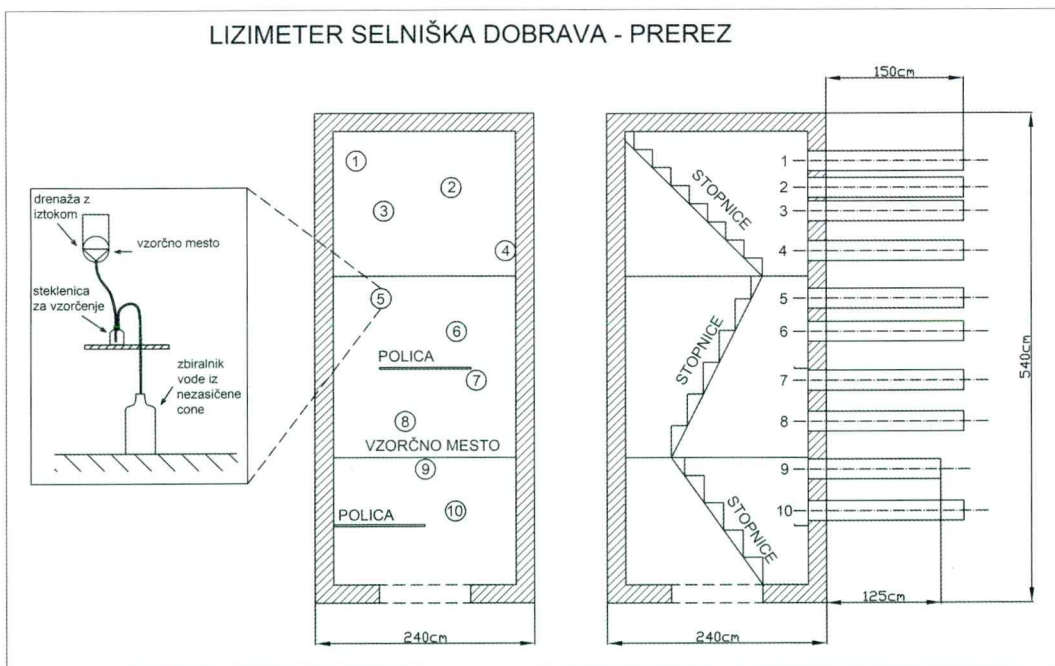
Sl. 2. Prerez lizimetra; lokacije vzorčnih mest od JV-1 do JV-10
