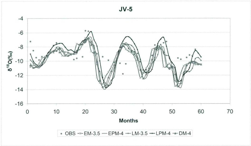
Sl. 7. Opazovane in prilagajane \delta^{18}\text{O} izstopne funkcije za vzorčno mesto JV-5 (modelirane vrednosti predstavljajo MRT v mesecih) Fig. 7. Observed and fitted \delta^{18}\text{O} output functions for sampling point JV-5 (model numbers present MRT in months)
