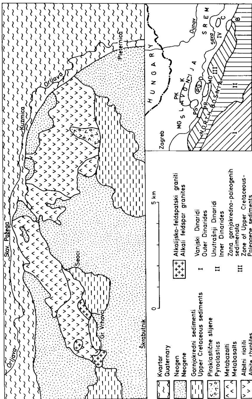
Sl. 1. Pregledna geološka karta sjevernih dijelova Požeške gore, po podacima Šparica i suradnici (1980) s tektonskom skicom dodirnog područja Dinarida i Panonskog bazena
