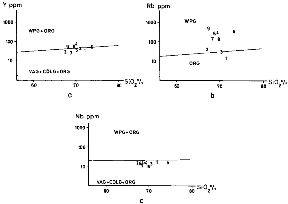
Sl. 6. Varijacioni dijagrami za Y (a), Rb (b) i Nb (c) u odnosu na SiO 2 (Pearce et al., 1984)
