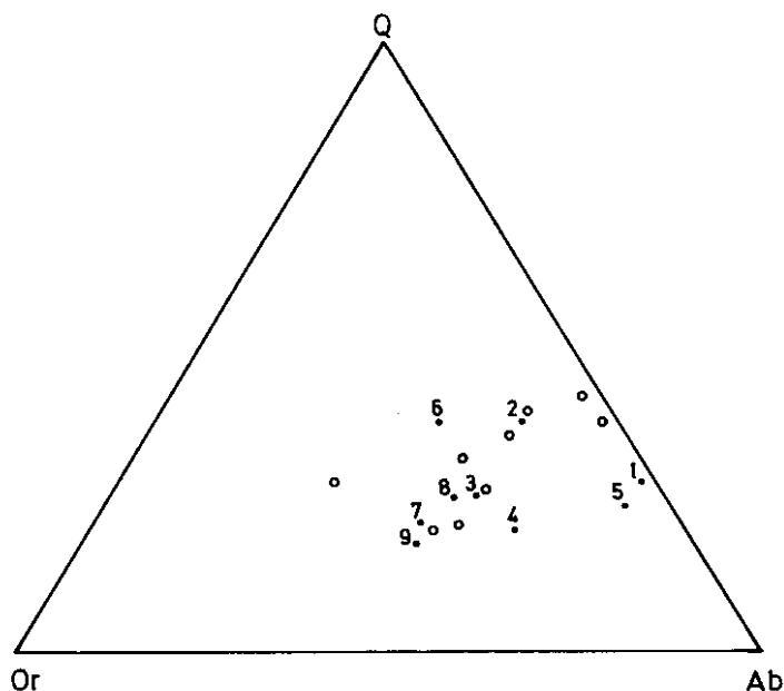
Sl. 5. Trokomponentni dijagram Q - Or - Ab za granite (označeni brojevima) i albitne riolite (označeni krugovima) Požeške gore
