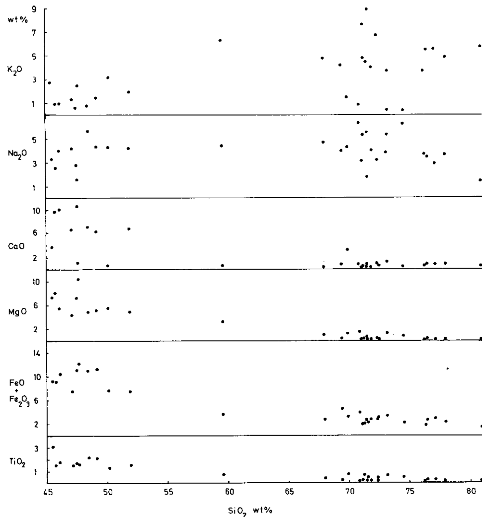
Sl. 5. Harkerovi dijagrami za vulkanske stijene Požeške gore
