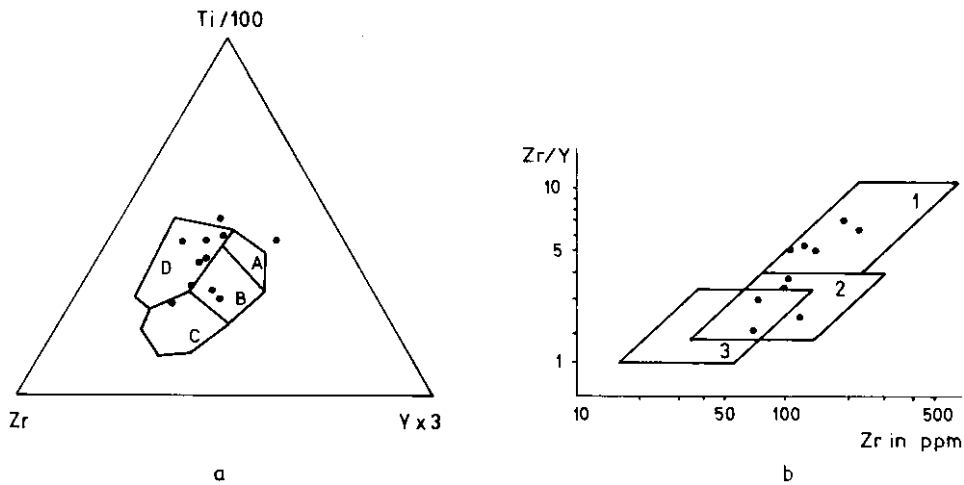
Sl. 6. a) Trokomponentni dijagram Ti:Zr:Y (Pearce & Cann, 1973), b) dvokomponentni dijagram Zr:Zr/Y (Pearce & Norry, 1979) A oceansko otočje; B abisalni toleiti; C bazalti otočnih lukova; D bazalti iz unutrašnjosti ploča Fig. a) Three component diagram Ti:Zr:Y (Pearce & Cann, 1973), b) Two component diagram Zr:Zr/Y (Pearce & Norry, 1979) A oceanic islands; B abyssal tholeiites; C island arc basalts; D within plate basalts
