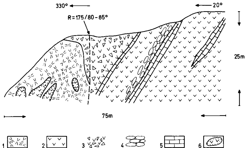
Sl. 2. Shematizirani geološki profil u kamenolomu Pako
