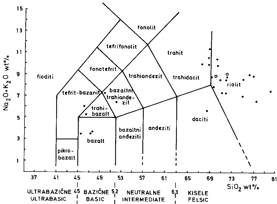
Sl. 3. Dijagram SiO 2 : Na 2 O + K 2 O (Le Bas et al., 1986)
