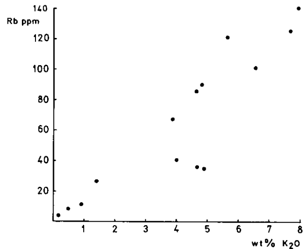
Sl. 7. Dijagram K_2O : Rb za alkalijsko-feldspatske riolite Fig. 7. The diagram K_2O versus Rb for alkali feldspar rhyolites
