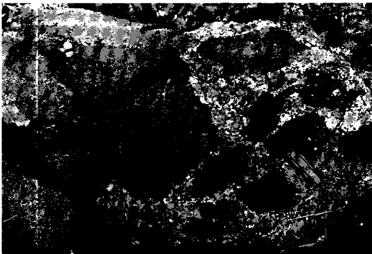
Sl. 4. Intruzivna magmatska breča. Nezaobljeni drobci mafičnega materiala v porfiroidnem granitu. Iz zadnjega prodirajo glinenci v mafične vključke (skrajni desni fragment)
