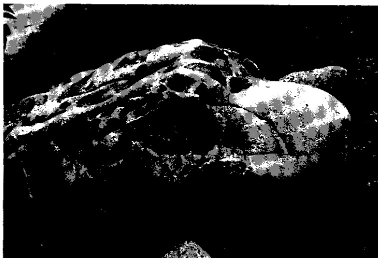
Sl. 2. Intruzivna magmatska breča. Drobnozrnati mafični magmatski vključki v porfiroidnem granitu. Oboje seče mlajša drobnozrnata granitna žila
