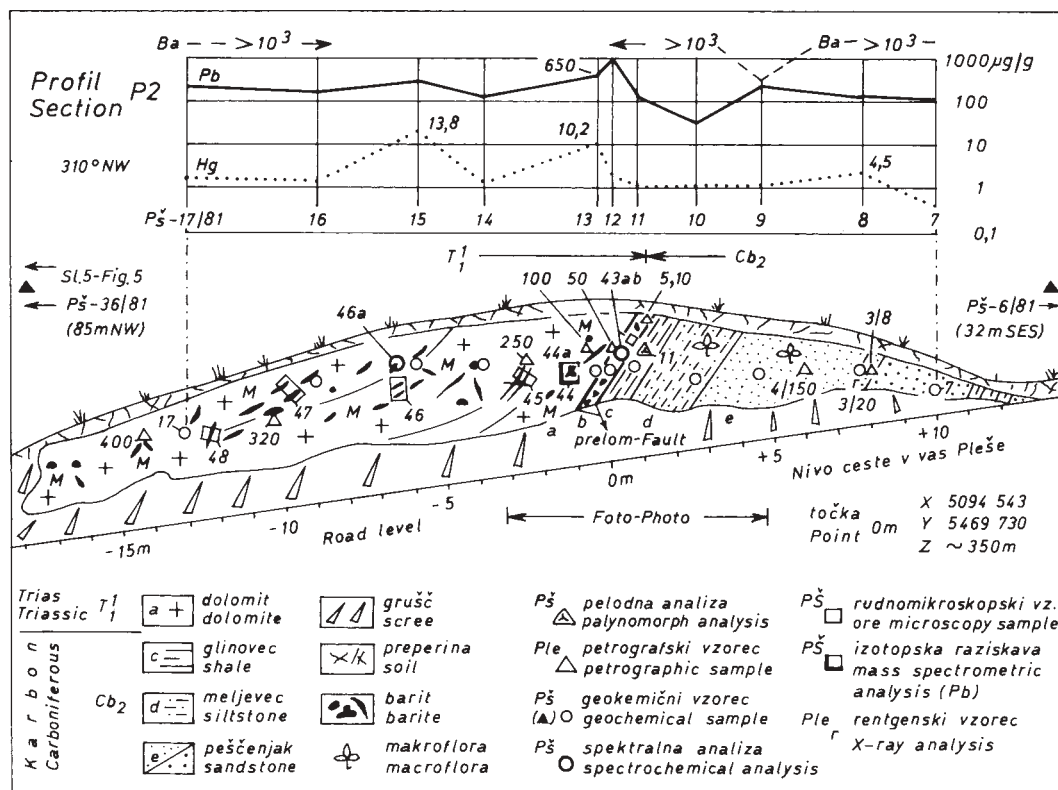
Sl. 4. Podrobno preiskani prerez P2 ob cesti v vas Pleše
