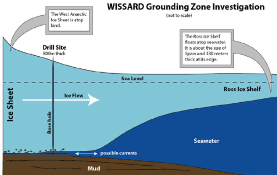
Sl. 12. Presek čez območje vrtnine SLW (Subglacial Lake Whillans) na ledeni plošči na zahodni Antarktiki (INTERNET 4).
