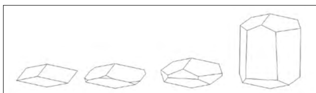
Sl. 12. Idealizirani kristali kalcita iz Liboj. Od leve proti desni sledijo: kalcit s kristalno formo položnega romboedra (012) in nato primeri z vedno bolj izraženimi kristalnimi formami strmega romboedra.
