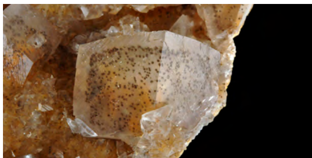
Sl. 13. Vključki manganovih oksidov in markazita so nastali po končani starejši fazi kristalizacije kalcita in so ujeti v mlajši fazi kristalov kalcita iz Liboj, 35 × 22 mm.
